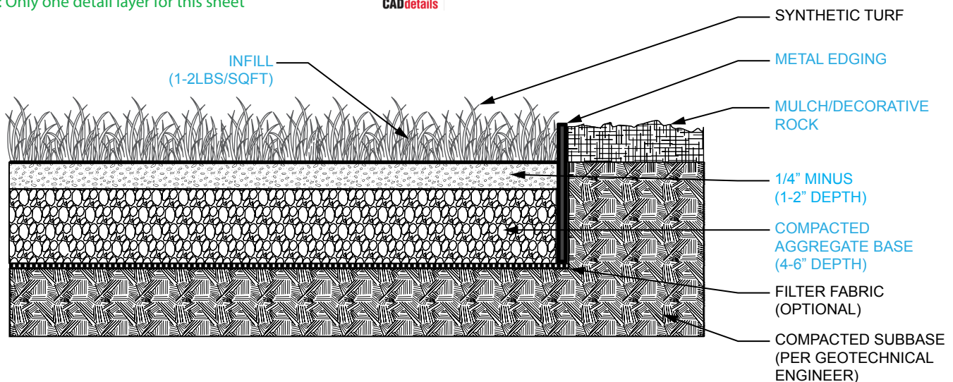
1 ENVYLAWN LANDSCAPE - METAL EDGE - DETAIL SCALE: NONE
